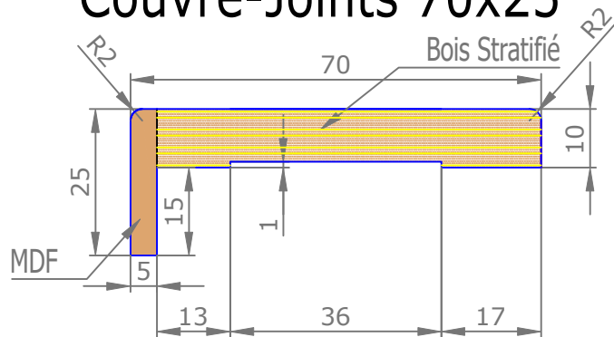
Couvre-Joints 70x25
