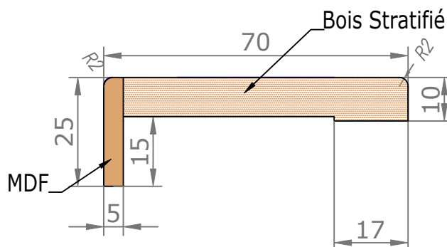
Couvre-Joints 70x25
