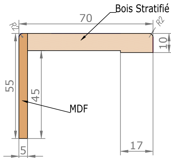
Couvre-Joints 70x55
