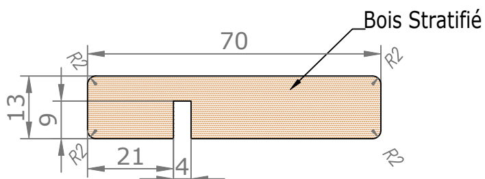
Couvre-Joints 70x13
