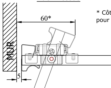
Tirant Droite
