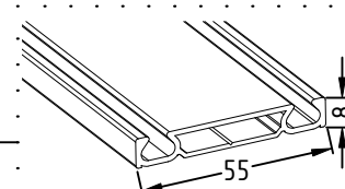
Rail Bas Alu laqué Finition : Anodisé ou laqué
