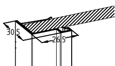
Profil Vertical : -Aluminium anodisé ou laqué
