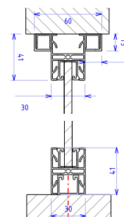
OPTION GRATUITE POSE BASSE SANS PARECLOSE
